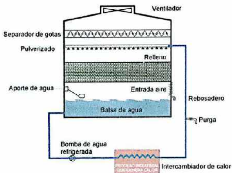
Figura 3. Representación del proceso de refrigeración (Ingenieriaviral 2022)
