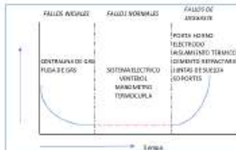
Figura 4: Curva de la bañera.
