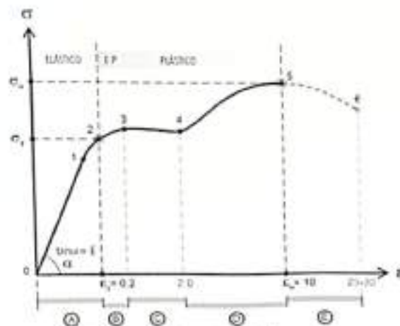
Ilustración 2: Etapas de Tensión-Deformación
