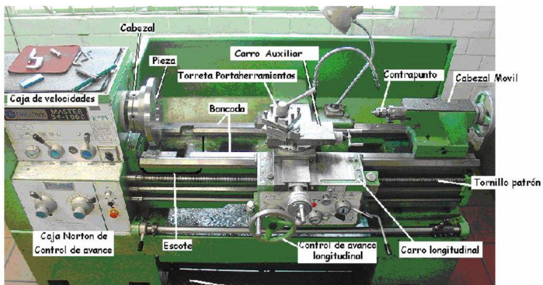
Figura 1. Partes principales de un torno horizontal
